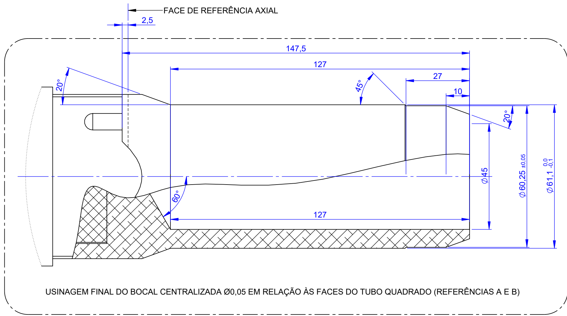
DETALHE H ESCALA 1 : 1
