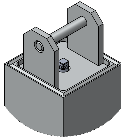
DETALHE G ESCALA 1 : 2
