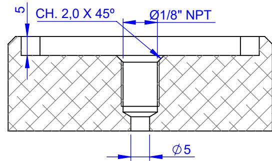
SEÇÃO E-E ESCALA 1 : 1
